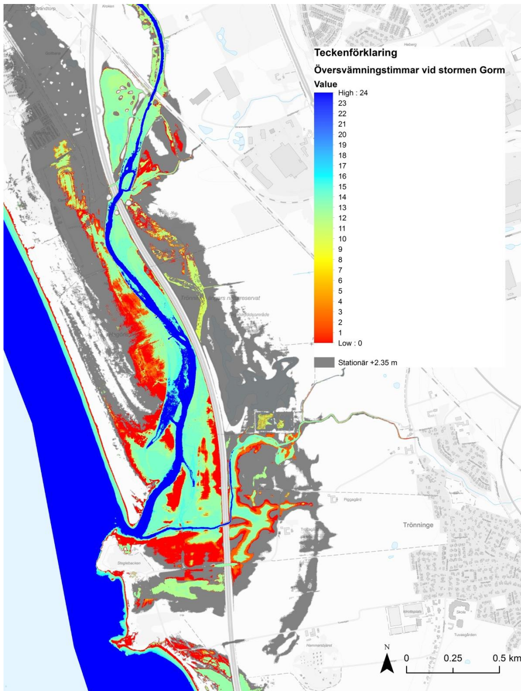
Figur 4 Antal timmar som mark översvämmas i samband med stormen Gorms händelseutveckling. Den grå ytan i kartan motsvarar översvämningsutbredning vid en stationär maxnivå på +2,35 m. Bakgrundskarta från Lantmäteriet.
